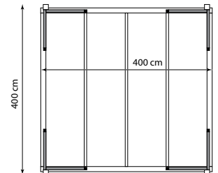
8 wand-elementen + 8 palen
