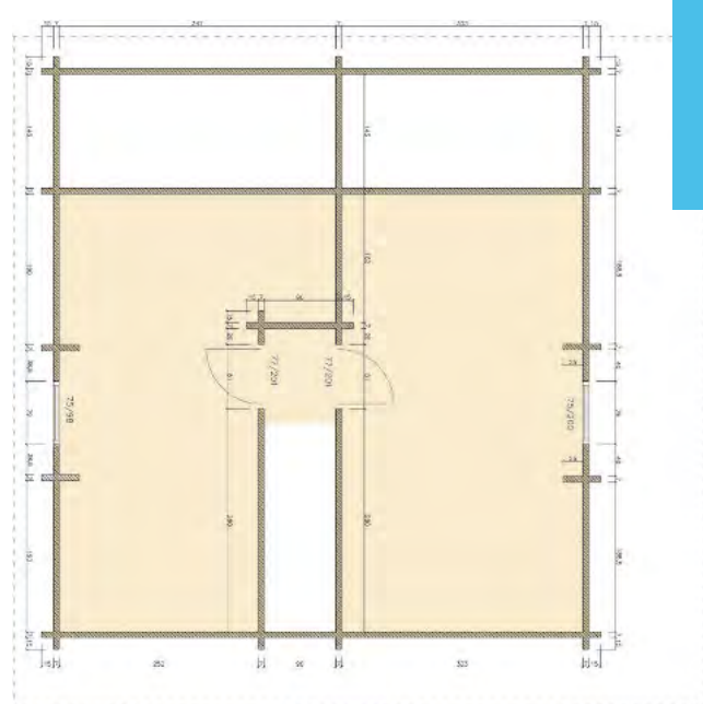
GRUNDRISS DG
